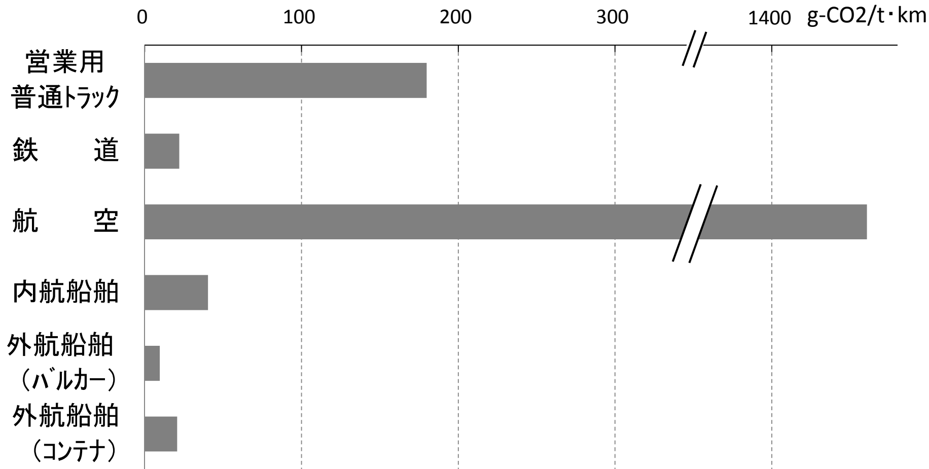
図4 輸送機関別に見た二酸化炭素排出係数
