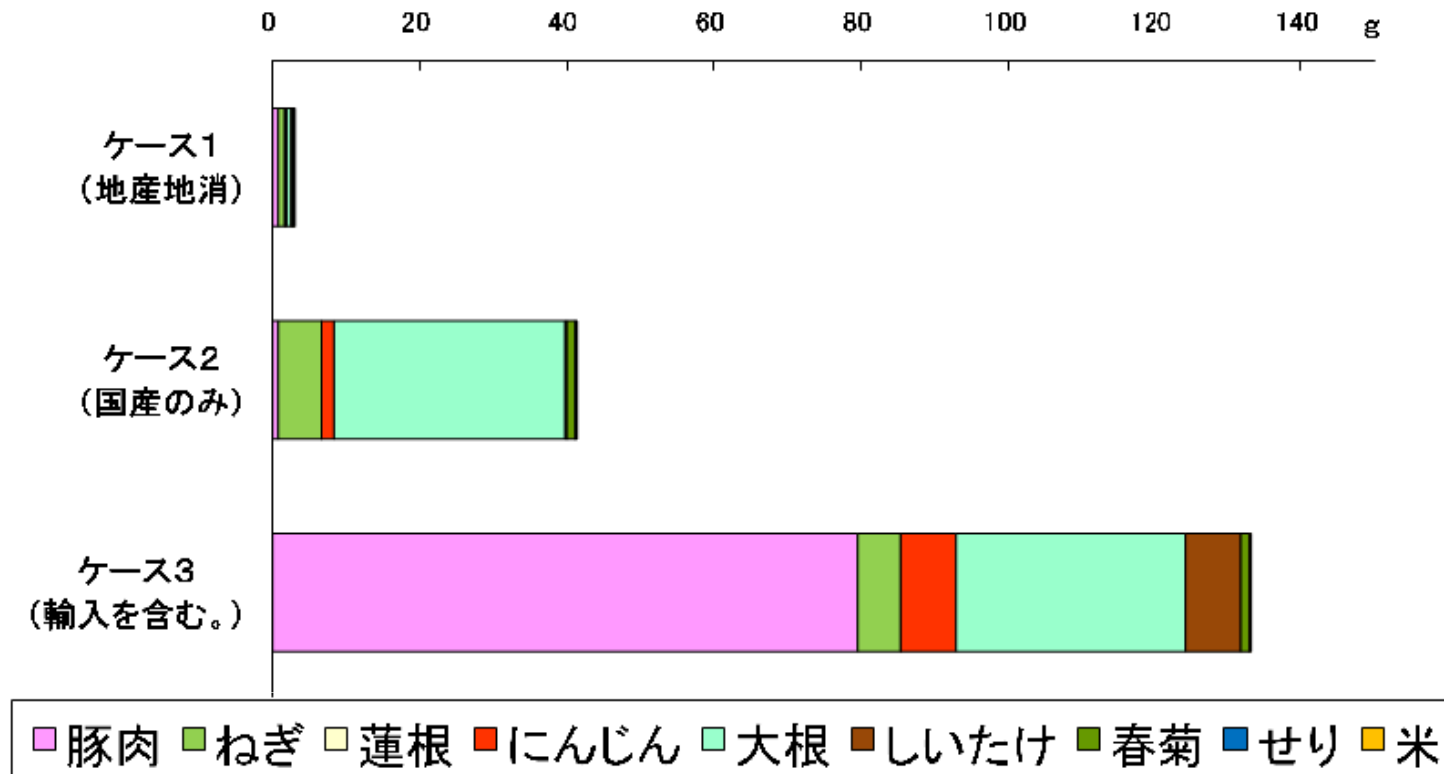
図8 ケーススタディ(加賀野菜等): 二酸化炭素排出量の比較
