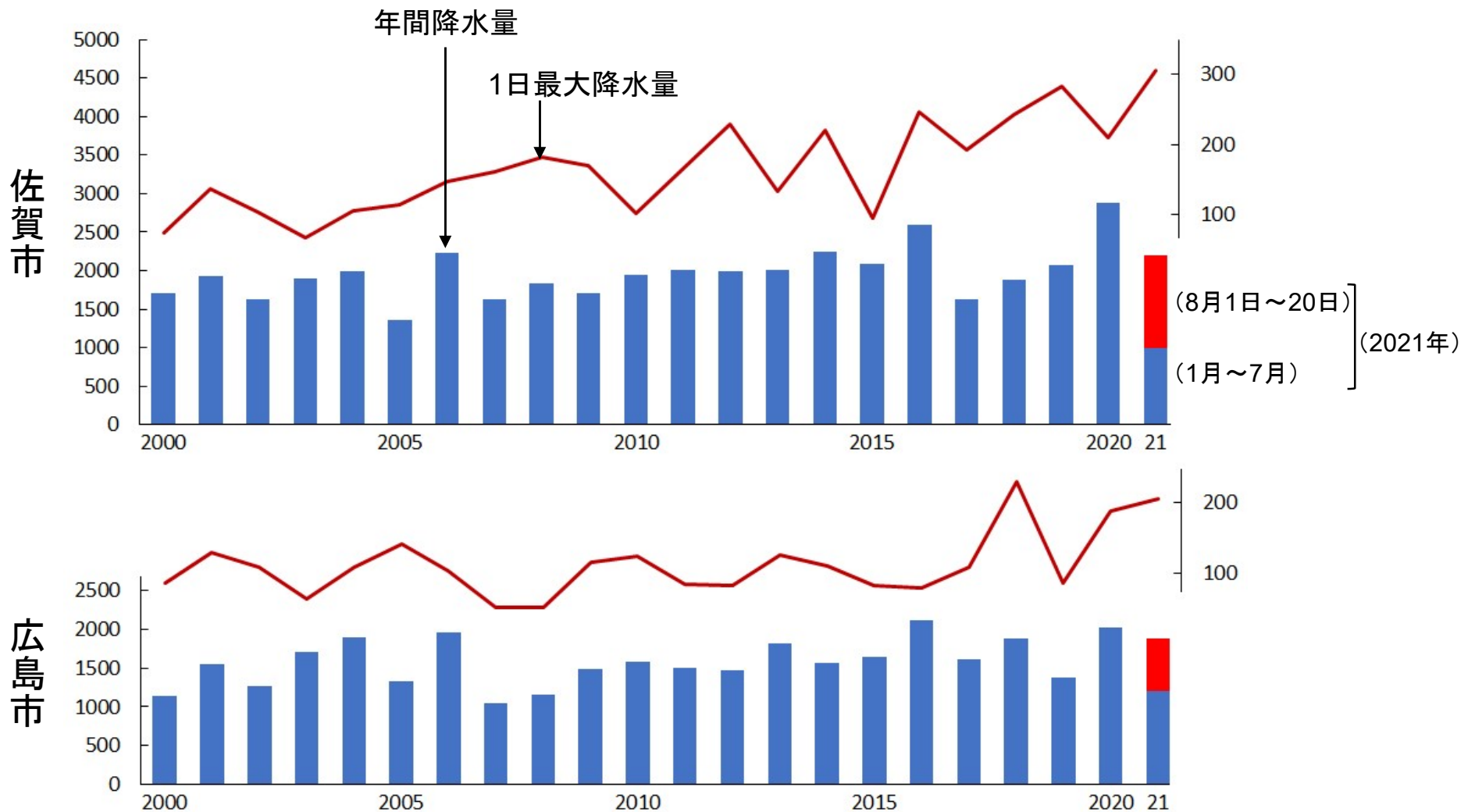
図224 年間降水量及び1日最大降水量の推移(佐賀市及び広島市)
